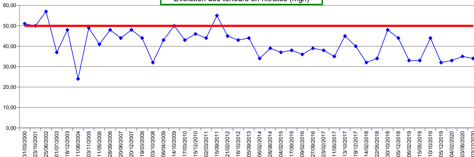
KERGAMET FORAGE 1. Evolution des teneurs en nitrates (mg/l)
